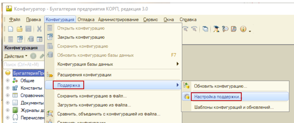
Рисунок 4 Настройка поддержки
