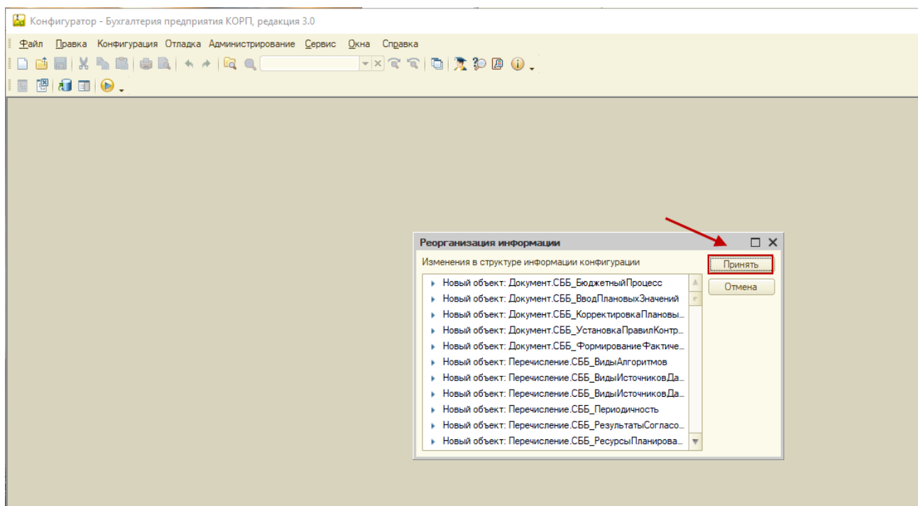
Рисунок 15 Реорганизация информации
