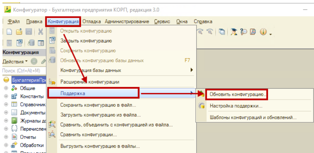
Рисунок 26 Обновление конфигурации
