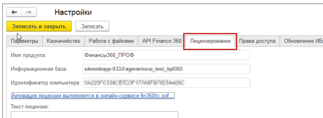
Рисунок 30 Настройки лицензирования
