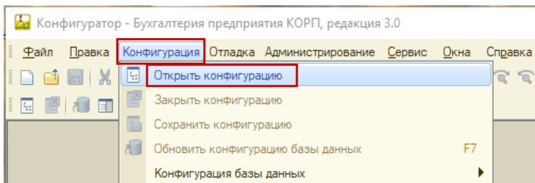
Рисунок 3 Открытие конфигурации
